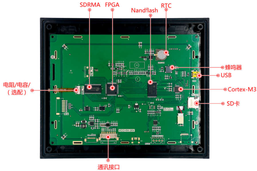
图 1-3 硬件配置图
