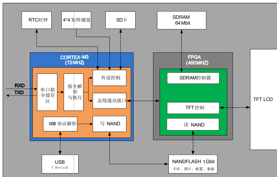
图 9-1 基本型串口屏内部结构图
