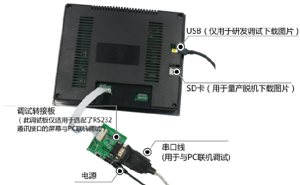
图 1-4 调试工具图
