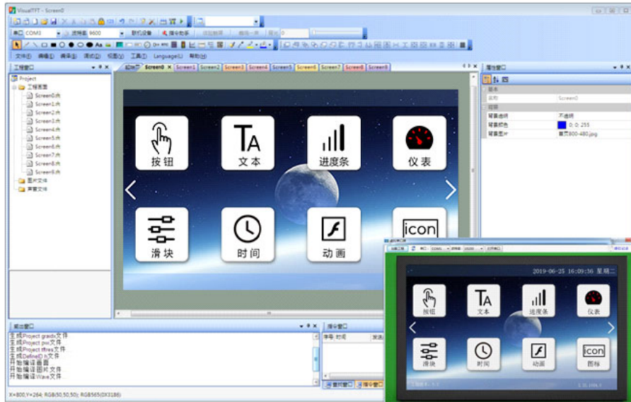
图 10-1 VisualTFT 主界面
